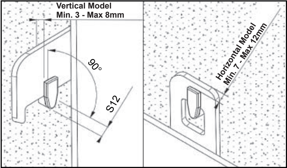
Schema di installazione - Installation scheme - Schéma d'installation - Esquema de instalación - Esquema de instalação - Schemat instalacji - Instalační schéma - Installationsschema - Montavimo schema - Instalācijas shēma - Paigaldamise juhend - Схема установки - Schemat instalacji - Instalacijski dijagram - Schema de instalare - Монтажна схема - مخطط التركيب - Kurulum şeması - Instalačná schéma - Dijagram instalacije - Instalacijska shema - Орнату схемасы - Installatieschema - Σύστημα εγκατάστασης - Схема установки
